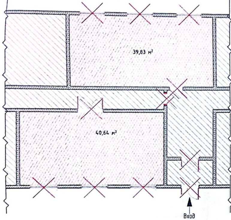
План демонтажа М1 : 100
